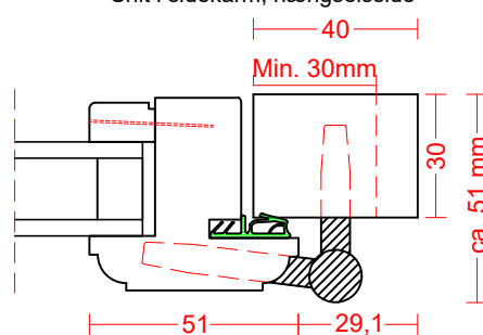
Snit i sidekarm, hængselsside
