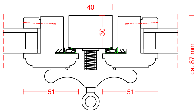
Snit i lodpost, anslagssider
