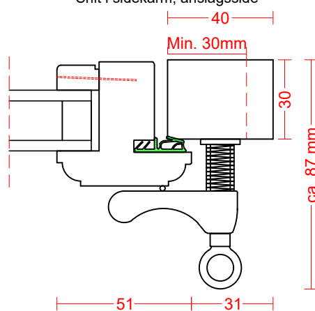
Snit i sidekarm, anslagsside
