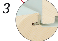
Der er ingen overfalsning på rammerne, og tætningslisten er skjult i karmen. Dermed ses ingen skyggekanter indefra.
