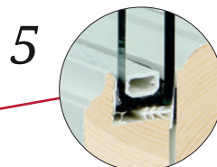
Diffusionsbånd reducerer rengøring mellem rammerne og giver en bedre lyd- og varme-isolering. Et Bøjsø Patent.
